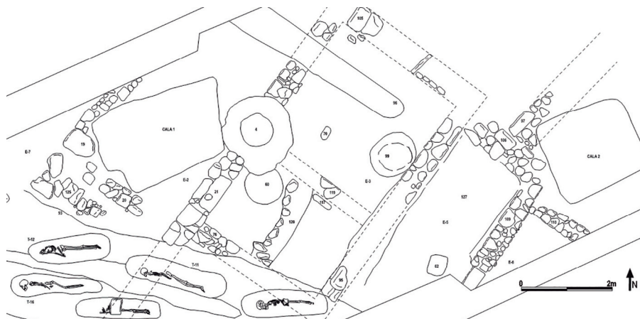
Figura 8. Planimetria de les estances a l'est del jaciment.
