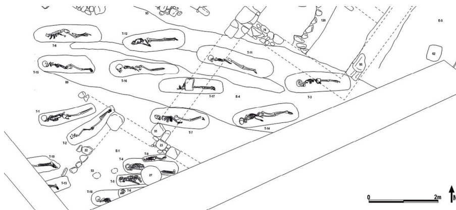
Figura 4. Planimetria de la màqbara.
